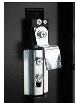
Zamek od strony wewnętrznej
